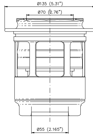
Montage sur réservoir Mounting on tank
